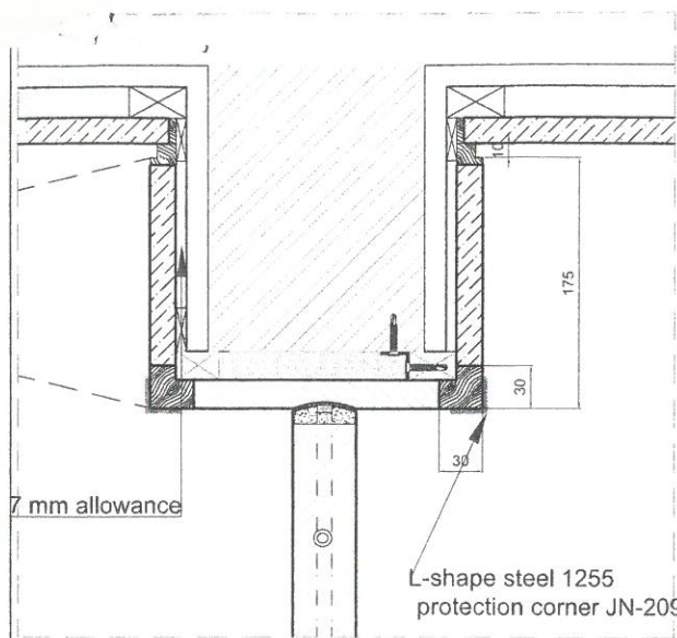
D1 Junction details
